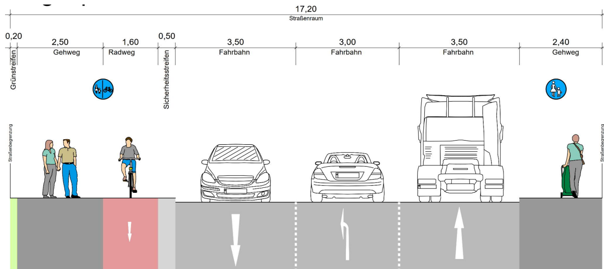
Abbildung 19 - Regelquerschnitt Lutzhorner Landstraße
