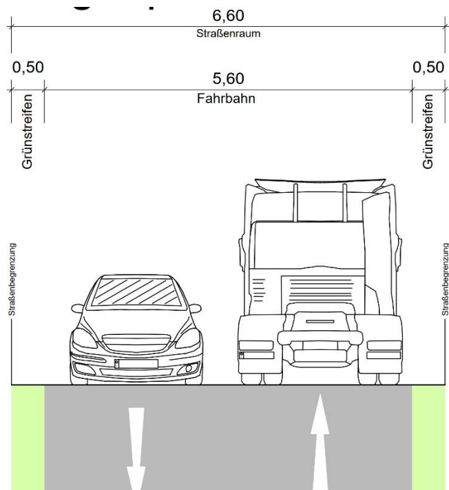
Abbildung 18 - Regelquerschnitt Knüppeldamm
